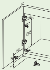
Wymiary montażowe Mounting dimensions / Монтажные размеры
