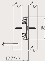
Wymiary montażowe Mounting dimensions Монтажные размеры
