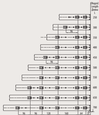
Pozycja mocowania prowadnik korpusu Fixing position of body slides Место крепления направляющей к корпусу
