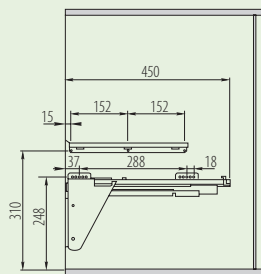
Rozstaw otworów montażowych prowadnicy i mocowania pokrywy Slide and cover mounting holes
