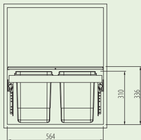
Wymiary gabarytowe / Dimensions / Габаритные размеры
