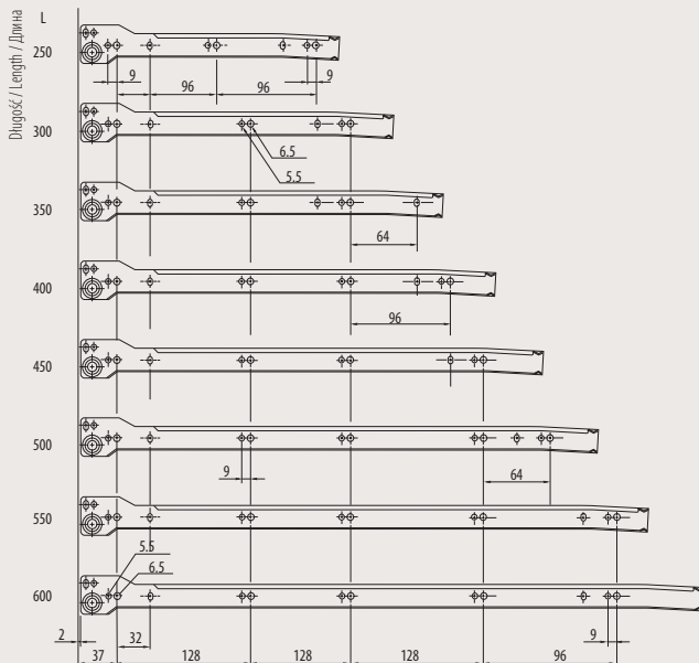
Schemat prowadnicy szuflady dla L=250 mm Drawer slide scheme for L=250 mm Схема направляющей ящика для L=250 mm
