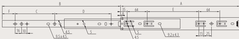
Wymiary montażowe Mounting dimensions Монтажные размеры
