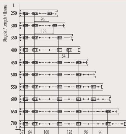
Pozycja mocowania prowadnic korpusu / Fixing position of body slides Место крепления направляющей к корпусу
