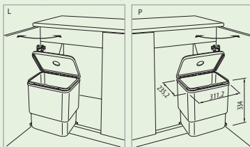
Sposób montażu Instruction of installation / Способ монтажа
