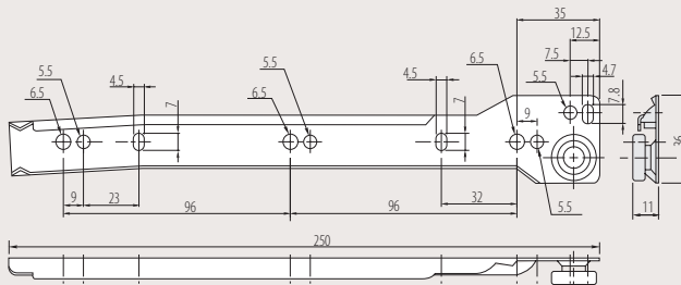
Schemat prowadnicy korpusu dla L=250 mm Body slide scheme for L=250 mm Схема направляющей корпуса для L=250 mm
