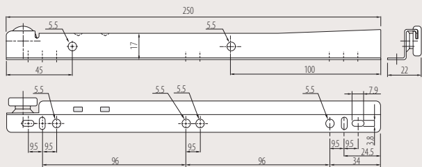
Schemat prowadnicy korpusu dla L=250 mm Body slide scheme for L=250 mm Схема направляющей корпуса для L=250 mm
