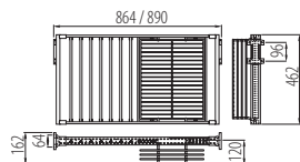
Wymiar wieszaka: 864 mm dla szafki L = 900 mm Hanger dimension: 864 mm for cupboard L = 900 mm Размеры вешалки 864 мм для шкафа L = 900мм
