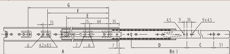
Pozycja mocowania prowadnic korpusu / Fixing position of body slides Место крепления направляющей к корпусу
